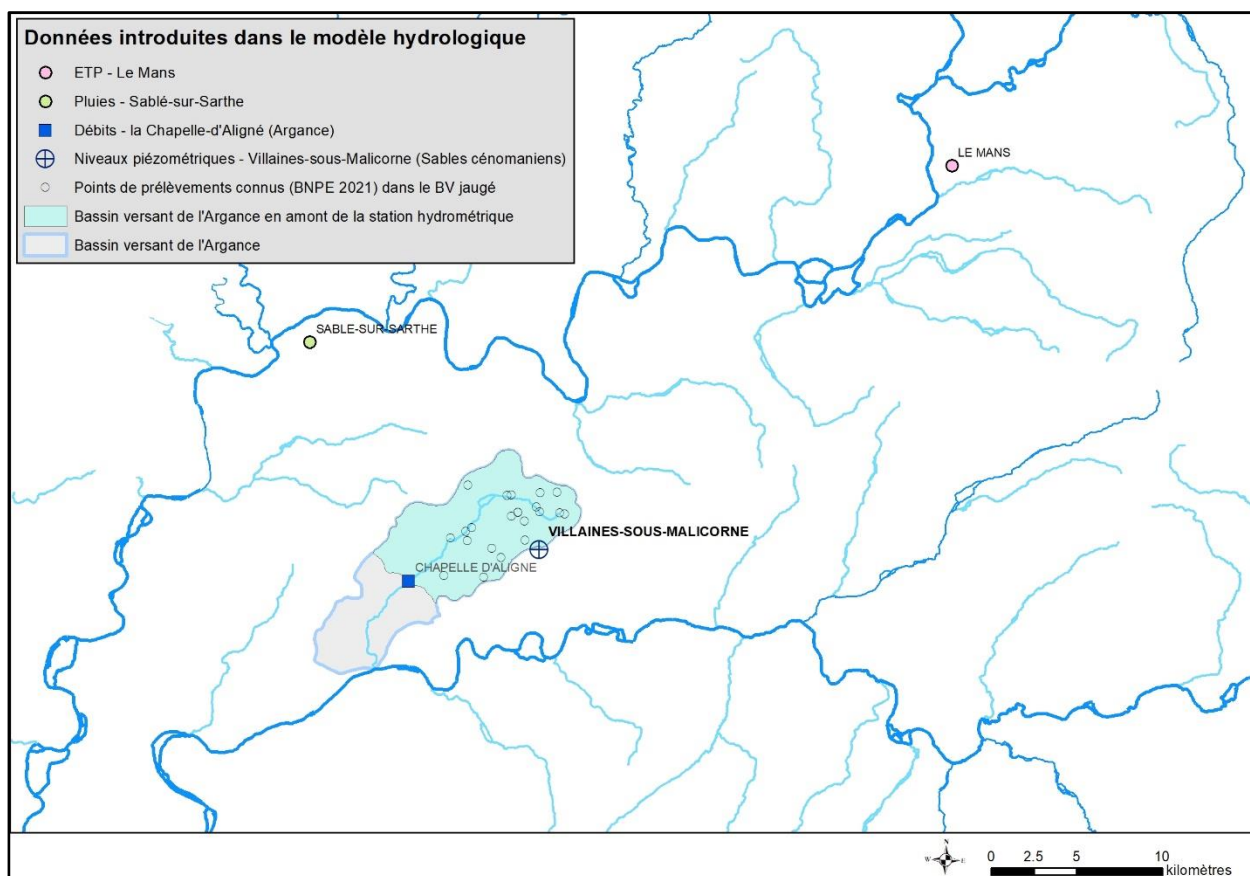
Illustration 4 : Localisation des stations de mesures dont les observations ont été introduites dans le modèle
