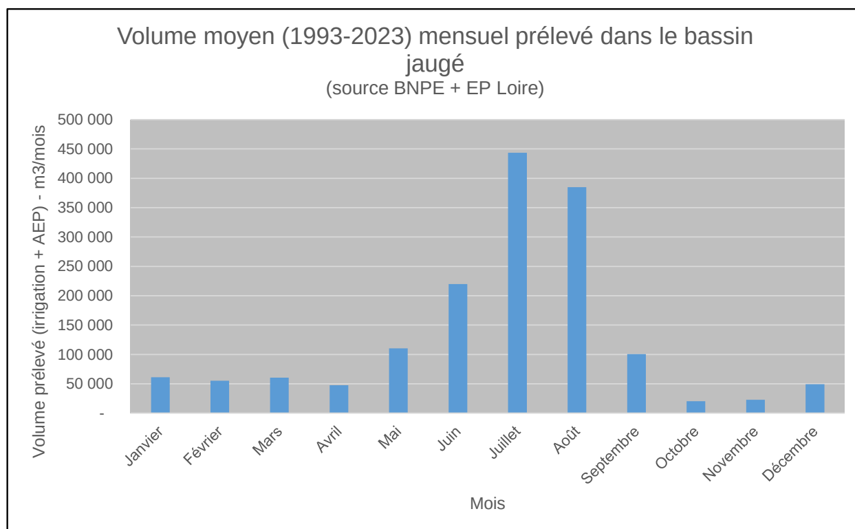
Illustration 6 : Prélèvements moyens mensuels intégrés dans le modèle global GARDENIA©
