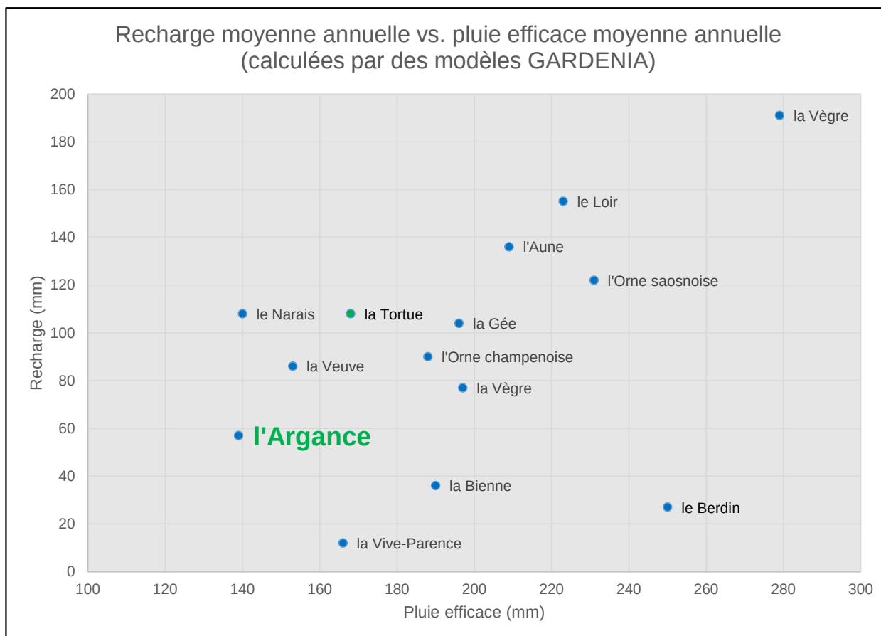
Illustration 13 : Recharge moyenne annuelle des nappes vs. pluie efficace moyenne annuelle.
