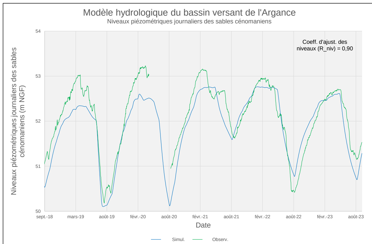
Illustration 10 : Ajustement des niveaux piézométriques des sables cénomaniens (détail des années 2016-2022).
