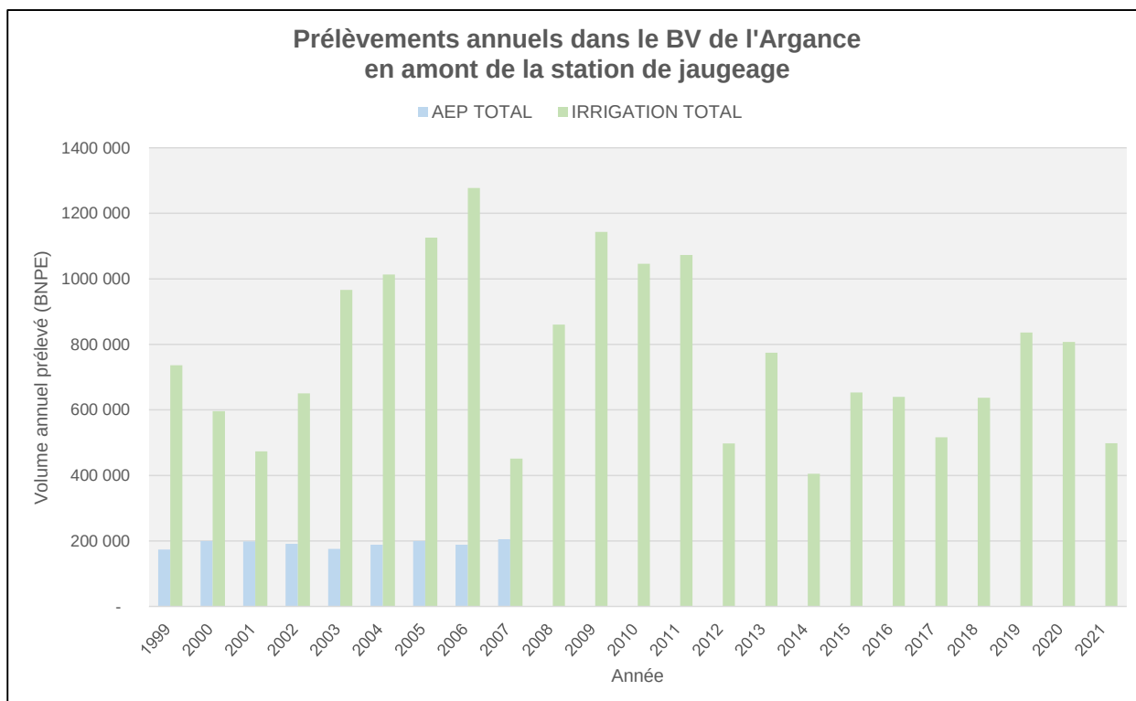
Illustration 5 : Prélèvements annuels connus dans le bassin versant de l'Argance en amont de la station hydrométrique entre 1999 et 2021 (BNPE).
