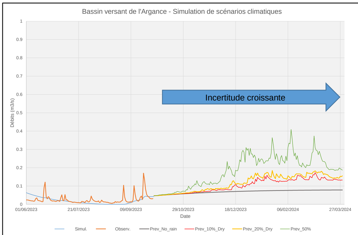
Illustration 16 : Prédiction des débits de l'Argance : zoom sur les plus faibles débits
