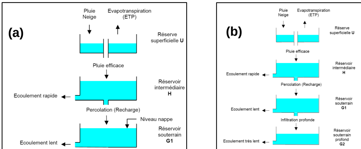
Illustration 3 : Schéma GARDENIA© à un seul réservoir souterrain (a) et deux réservoirs souterrains (b).
