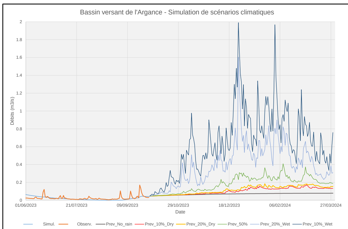
Illustration 15 : Prévision des débits de l'Argance (avec procédure adaptative).
