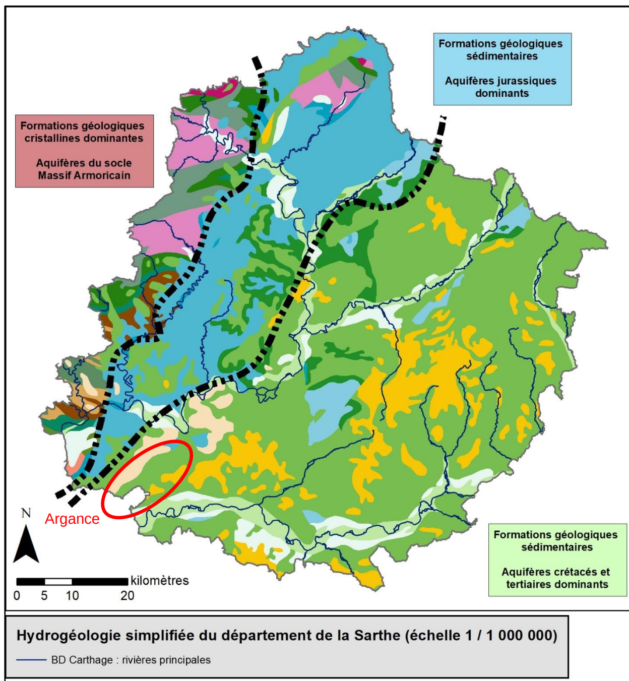
Illustration 1 : Hydrogéologie générale simplifiée du département de la Sarthe.
