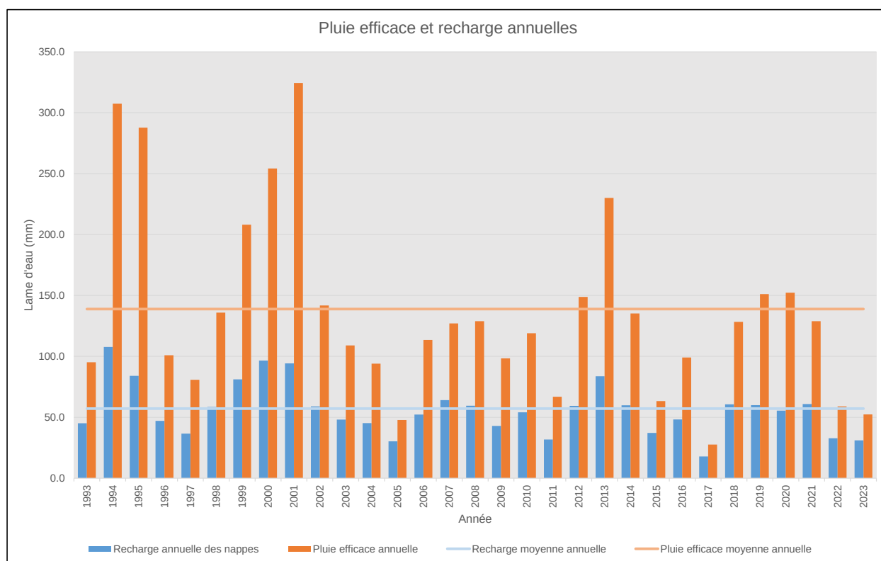
Illustration 11 : Pluie efficace et recharge annuelles.
