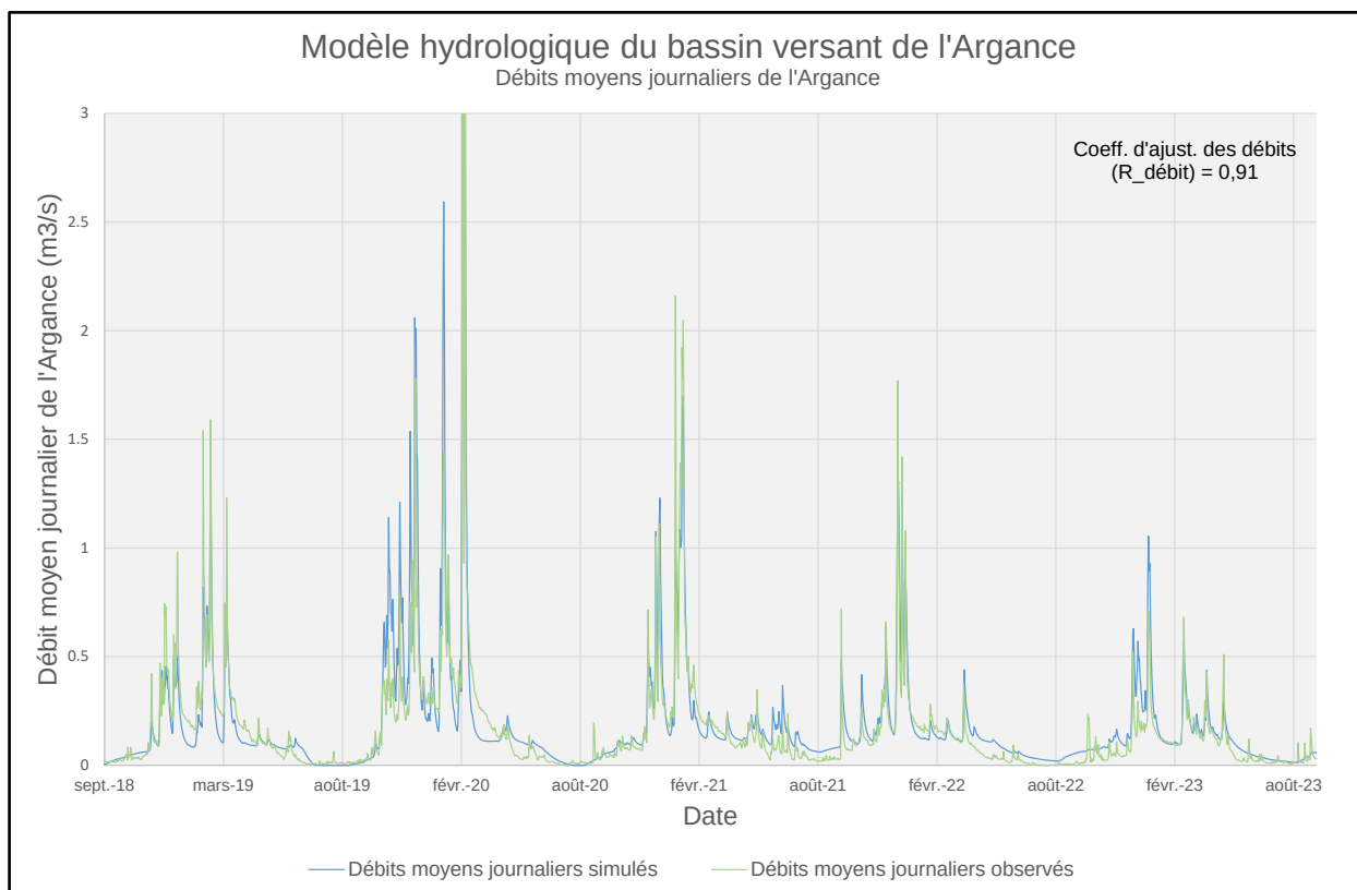
Illustration 8 : Ajustement des débits de l'Argance (détail des années 2016-2022).
