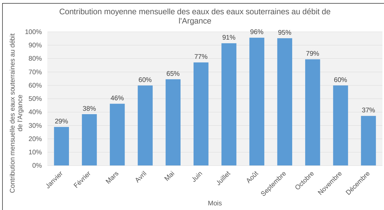
Illustration 14 : Histogramme de la contribution moyenne mensuelle des eaux souterraines au débit de l'Argance.
