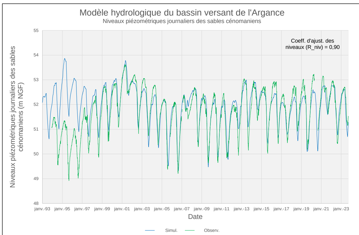
Illustration 9 : Ajustement des niveaux piézométriques des sables cénomaniens.
