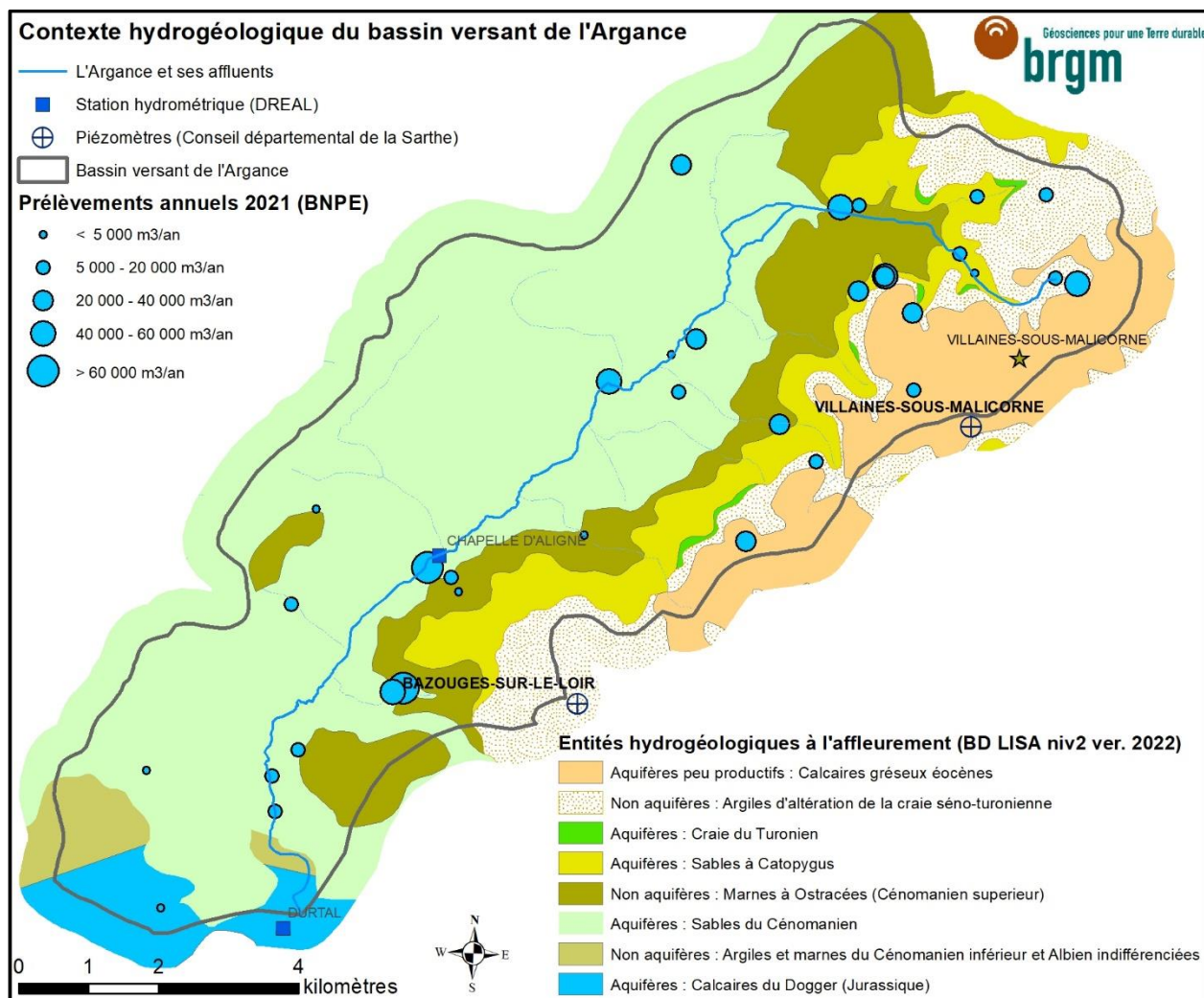
Illustration 2 : Contexte hydrogéologique simplifié du bassin versant de l'Argance.
