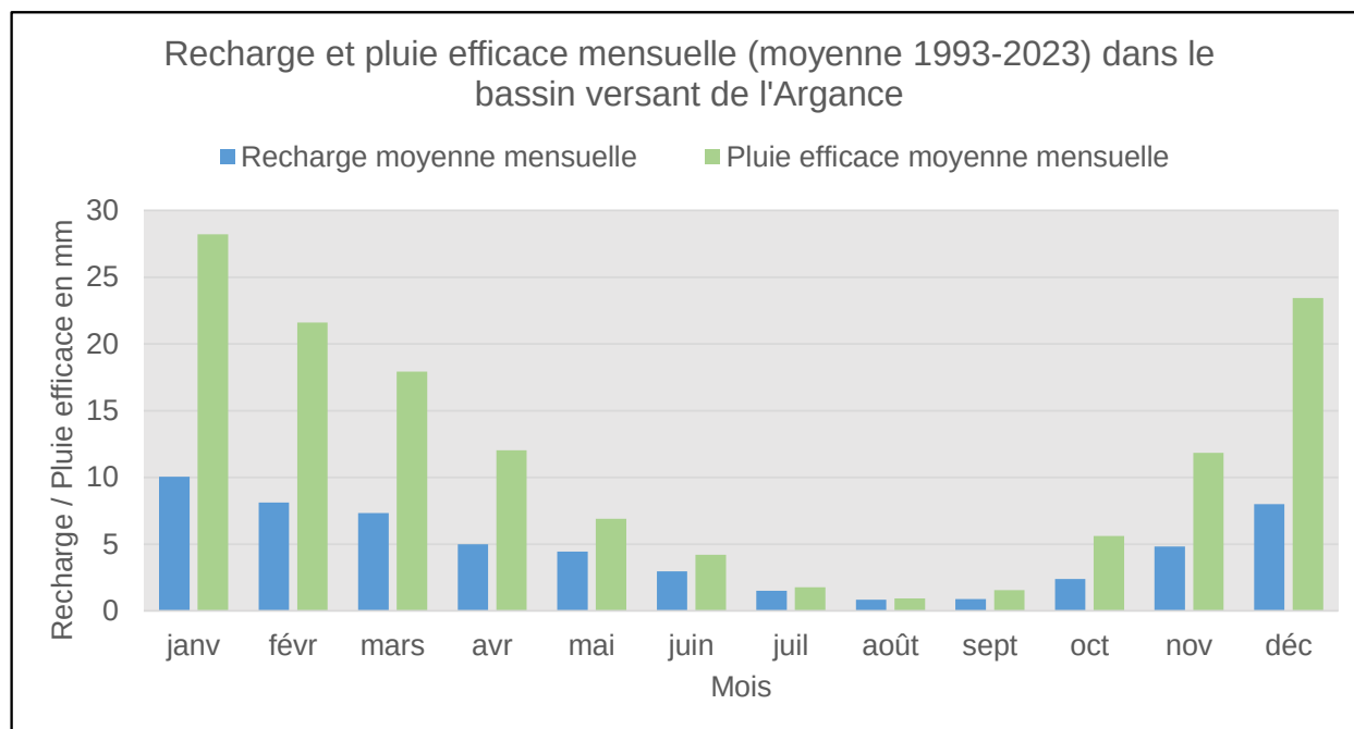
Illustration 12 : Recharge et pluie efficace mensuelle (moyenne 1993-2023).
