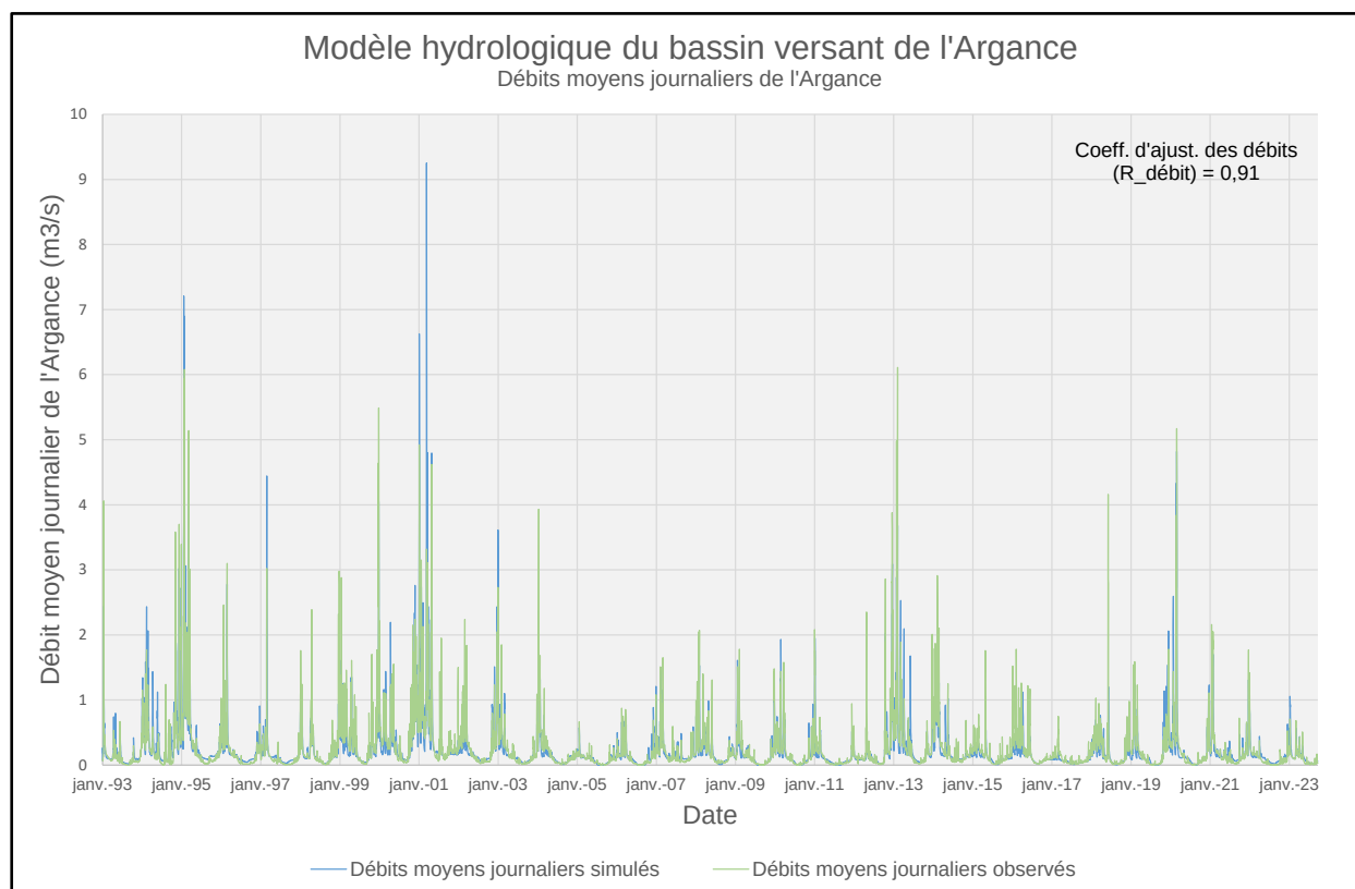
Illustration 7 : Ajustement des débits de l'Argance.
